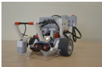
ROBOT LEGO MINDSTORM
